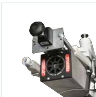
Groupe toupie T-M Pour l'exécution de rainures sur le côté supérieur du panneau.
