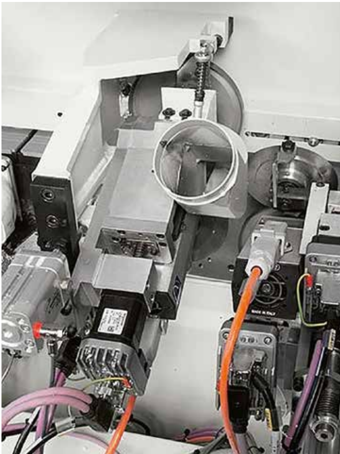
RAS-HP Multiedge 2R: 2 rayons différents sur les chants en plastique
