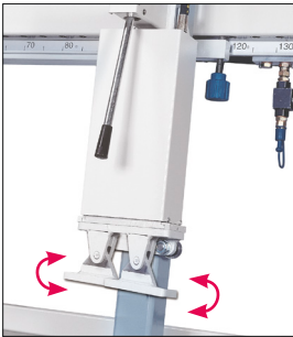
cylindres. Pieds de poussée articulés pour châssis inclinés.
